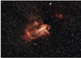
Photo de la Nébuleuse M17 avec un temps de pose d'une heure.
